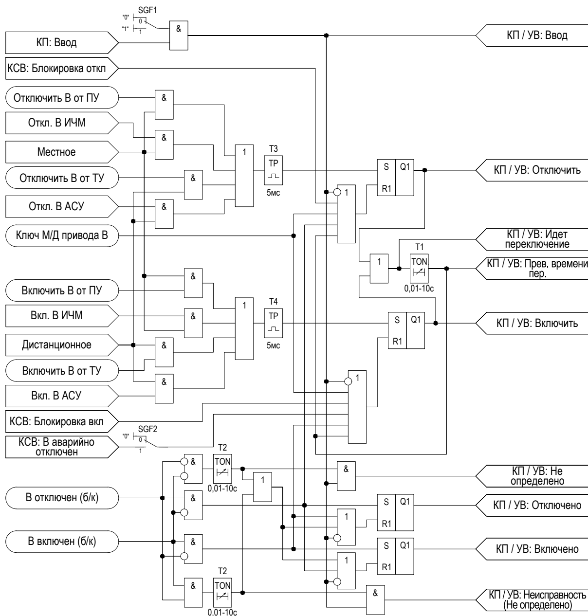
Рисунок 2.32 – Функциональная схема «УВ»
