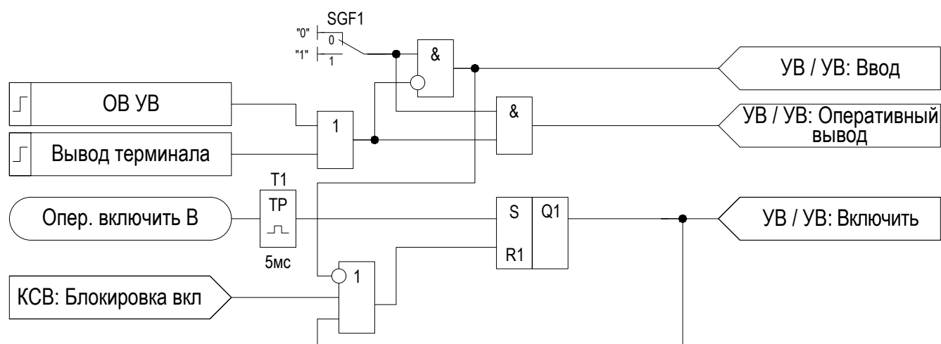
Рисунок 2.33 – Функциональная схема «УВ»
