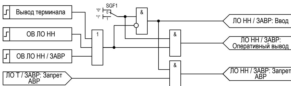
Рисунок 2.27 – Функциональная схема «Запрет АВР»
