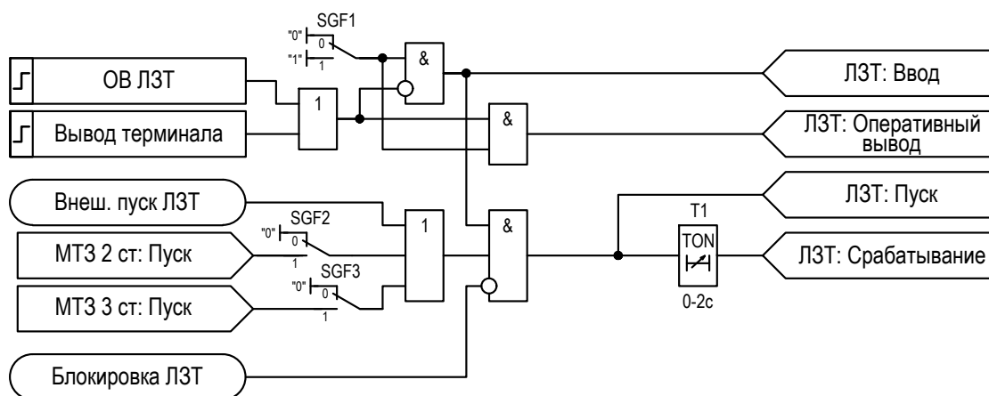
Рисунок 2.6 – Функциональная схема «ЛЗТ»
