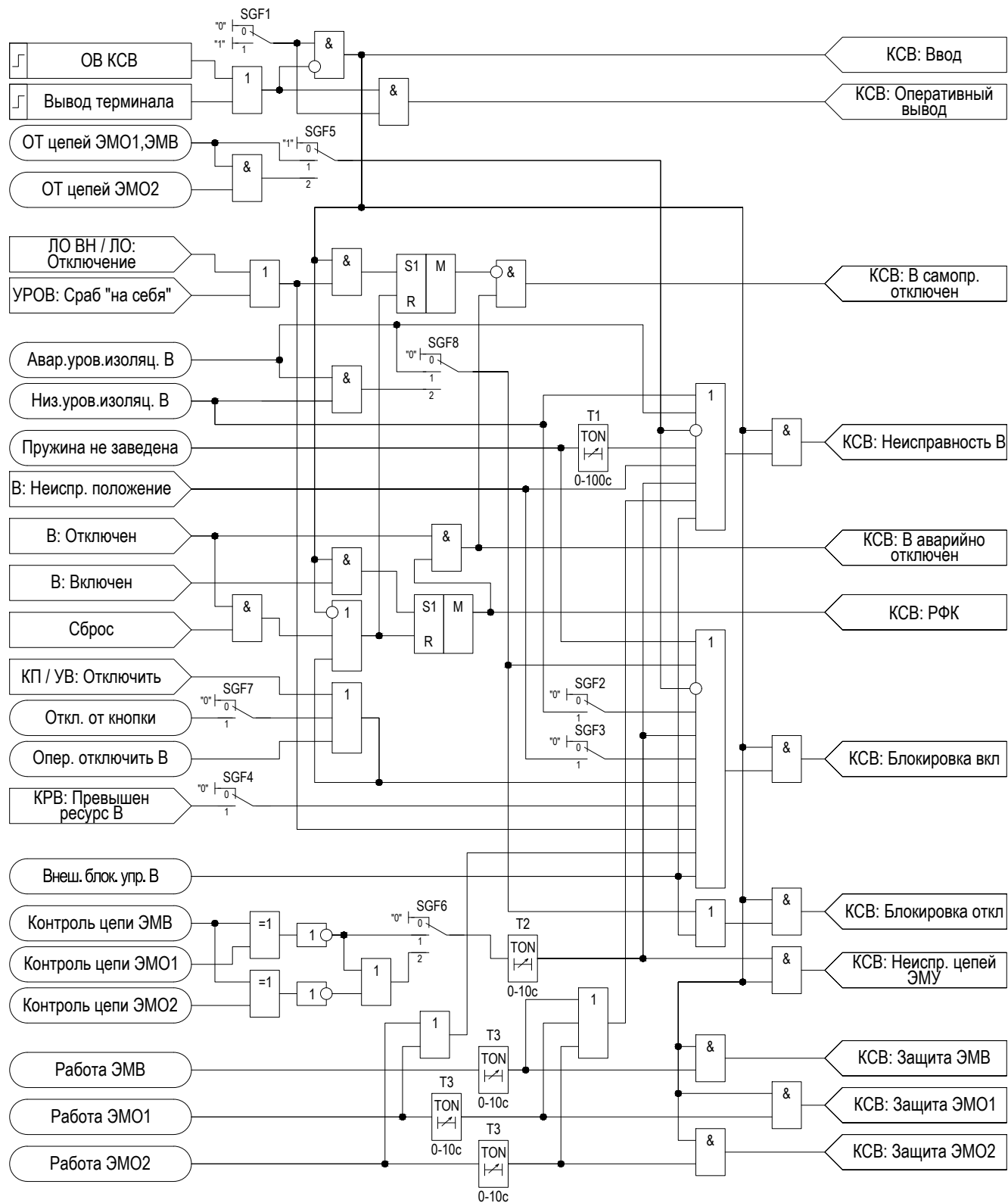
Рисунок 2.30 – Функциональная схема «КСВ»
