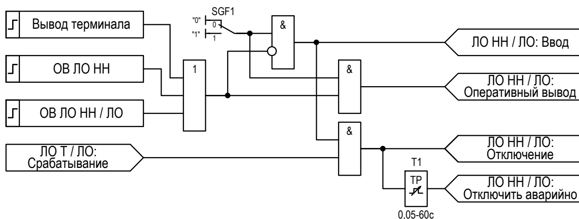
Рисунок 2.25 – Функциональная схема «ЛО»
