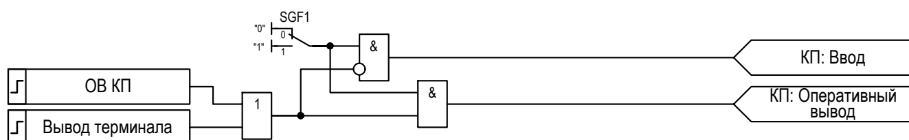
Рисунок 2.31 – Функциональная схема управления режимами работы «КП»
