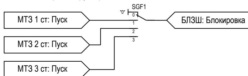
Рисунок 2.4 – Функциональная схема БЛЗШ
