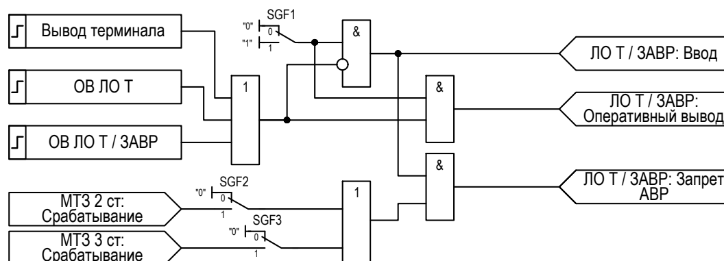
Рисунок 2.23 – Функциональная схема «ЗАВР»
