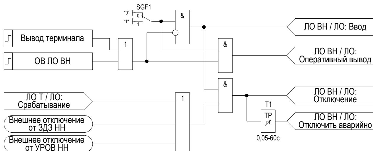
Рисунок 2.24 – Функциональная схема «ЛО»
