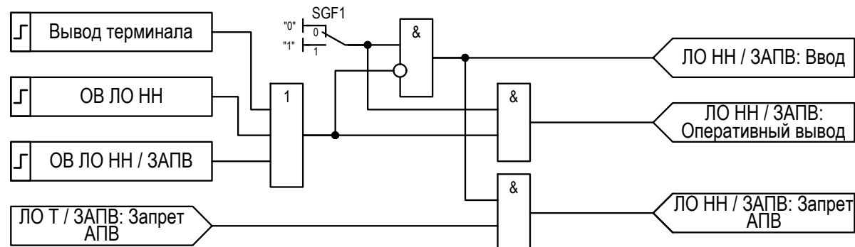
Рисунок 2.26 – Функциональная схема «Запрет АПВ»
