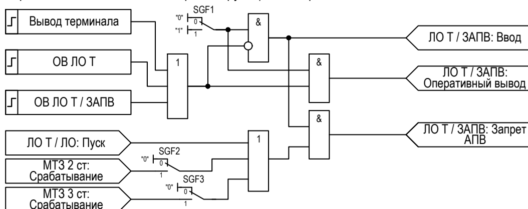
Рисунок 2.22 – Функциональная схема «ЗАПВ»
