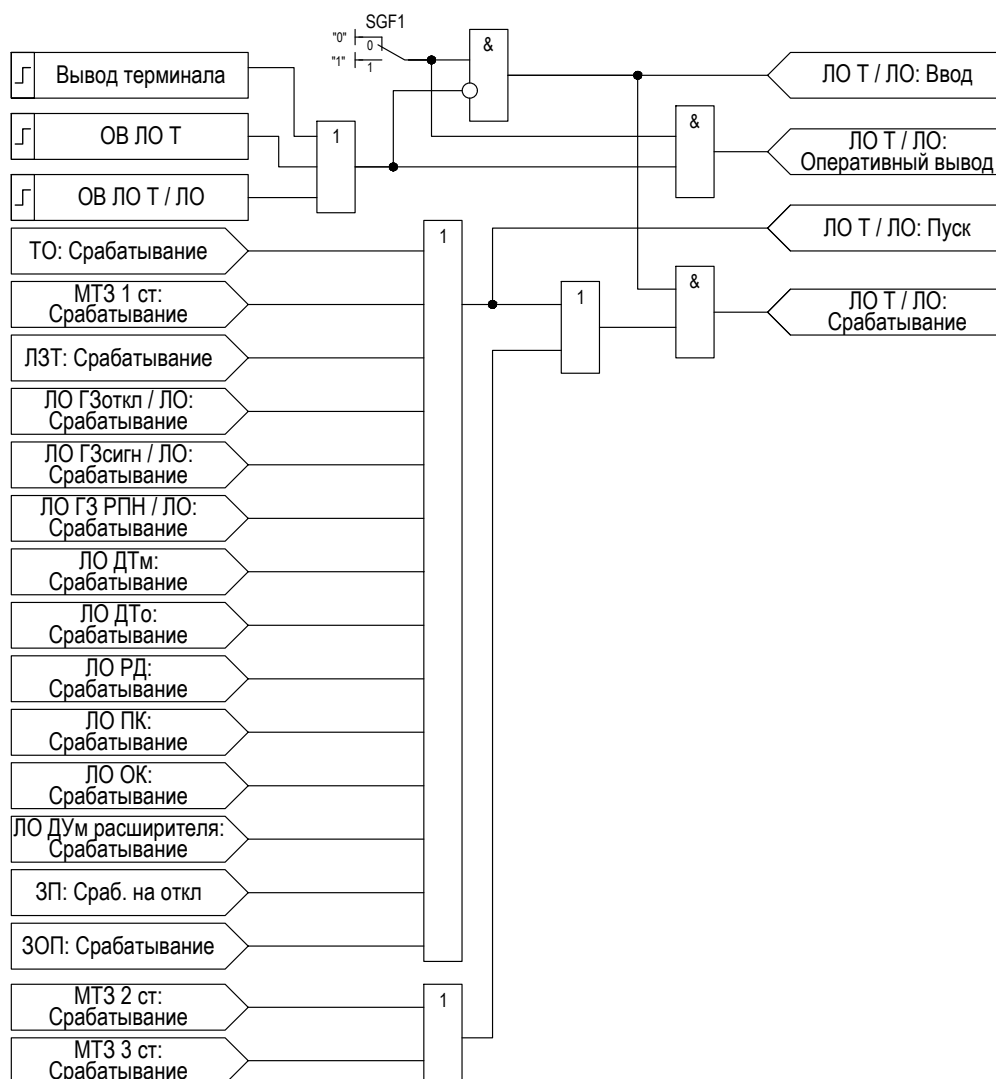
Рисунок 2.21 – Функциональная схема «ЛО»
