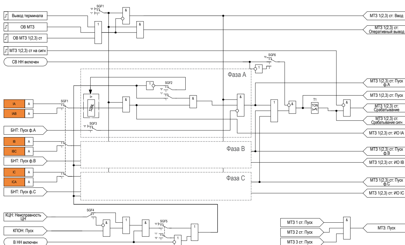
Рисунок 2.1 – Функциональная схема ступеней «MT3 1 ст», «MT3 2 ст», «MT3 3 ст»
