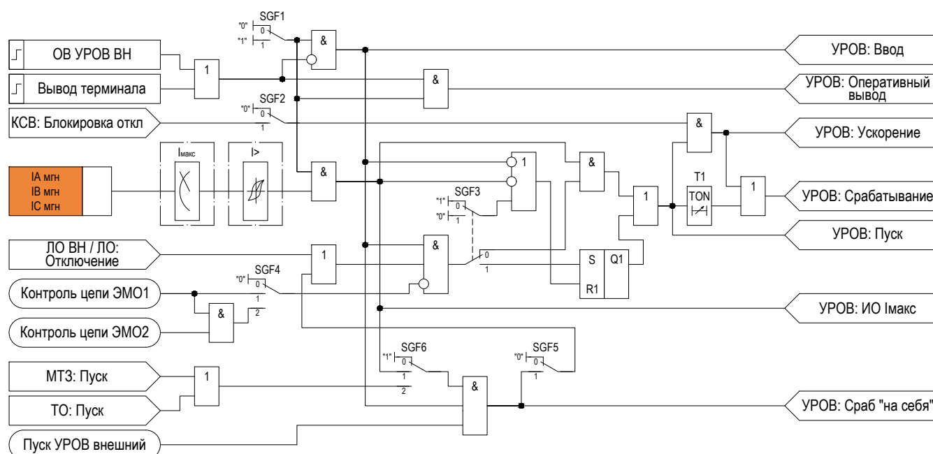
Рисунок 2.28 – Функциональная схема «УРОВ»
